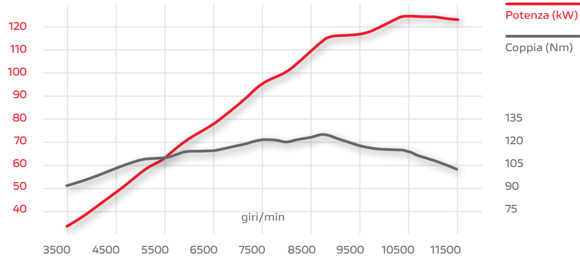
Curve di potenza / coppia
