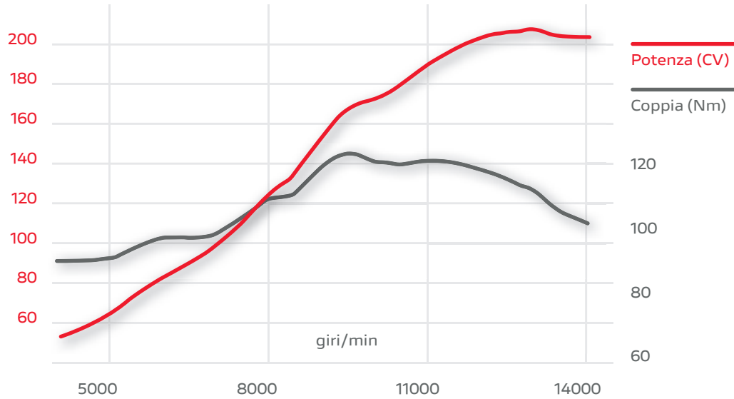
Curve di coppia / potenza
