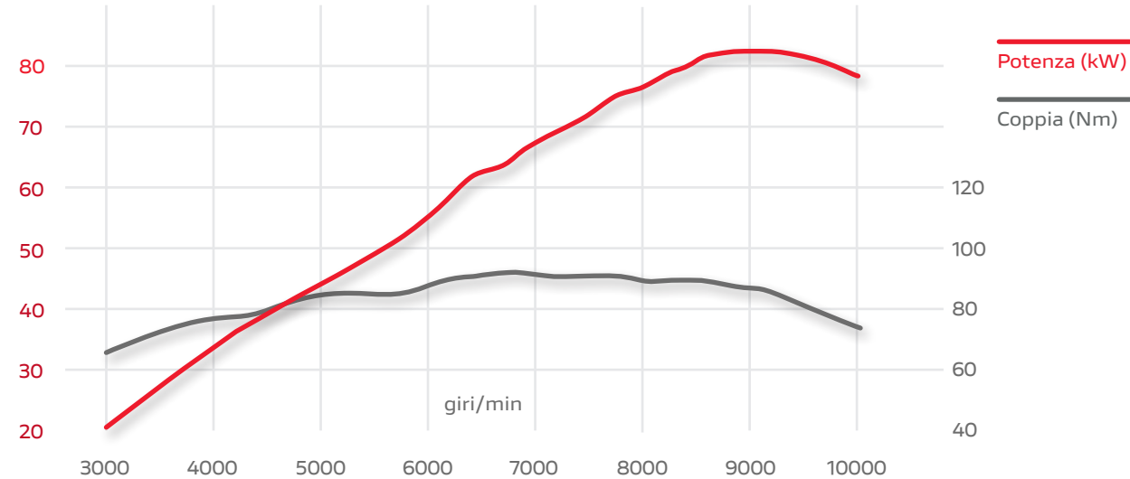
Curve di potenza / coppia
