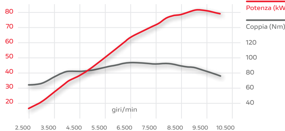
Curve di potenza / coppia
