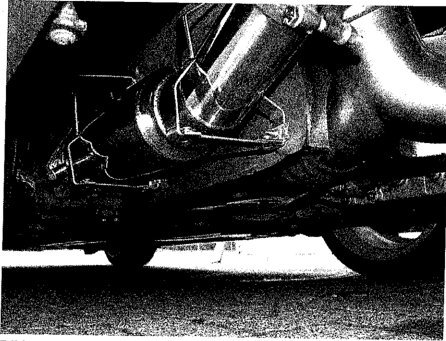
Ansicht Edelstahlkatalysator
