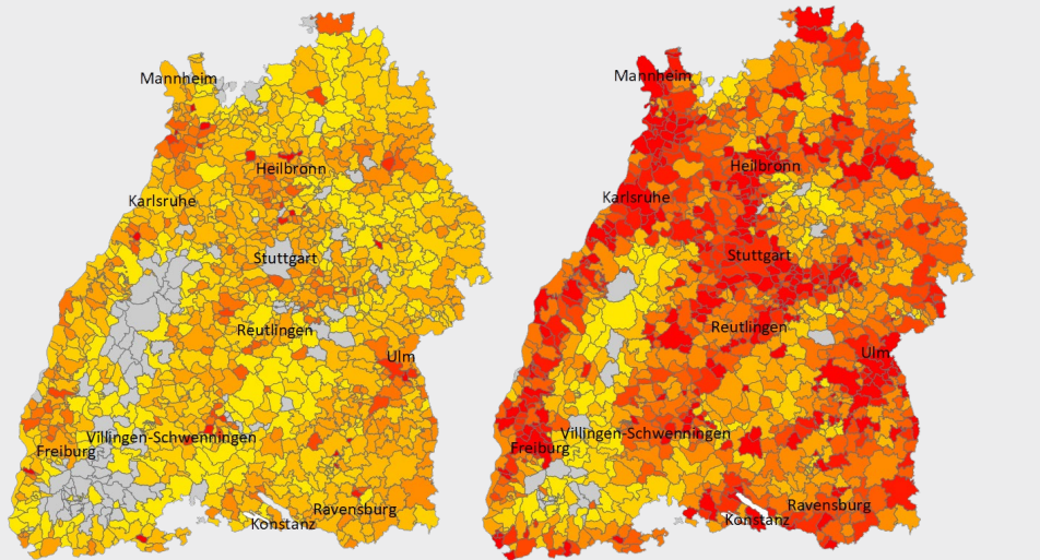
Abbildung 2: Verteilung der installierten und für 2035 prognostizierten Leistung an PV
