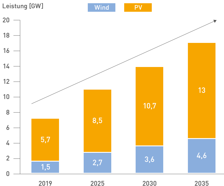
Abbildung 1: Interpolierter Hochlauf von PV und Windkraft bis zum Zielwert aus dem NEP [2]
