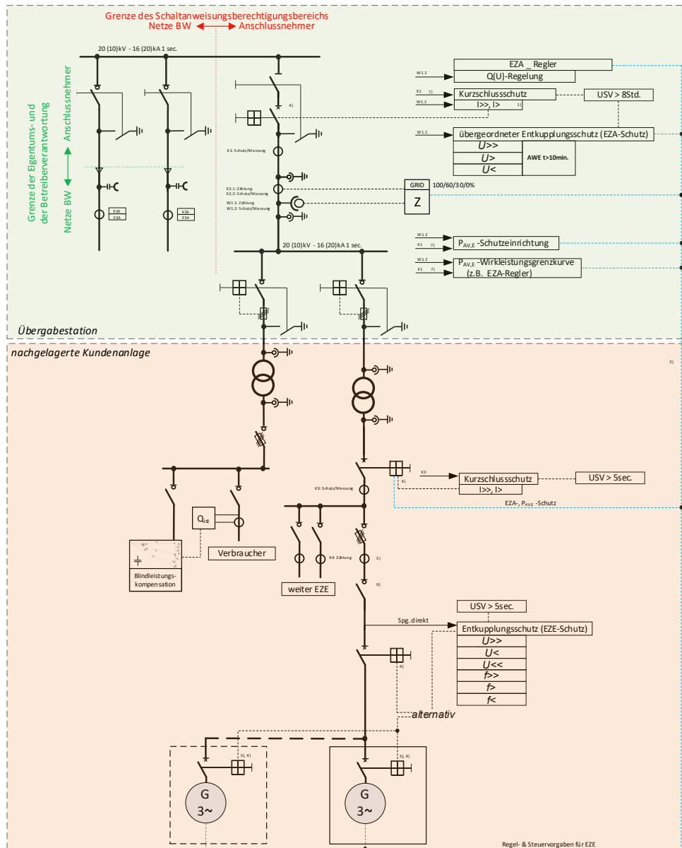
Bild D. 9: Misanlage mit Übergabeleistungsschalter und separatem Transformator mit Sicherungslasttrennschalter für die Erzeugungsanlage ( \sum EZA \leq 950 \text{ kW} )
