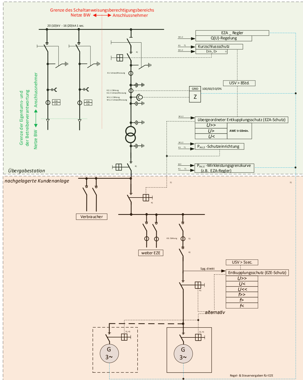
Bild D. 8: Mischanlage mit Leistungsschalter ( \Sigma E_{ZA} \leq 950 \text{ kW} )
