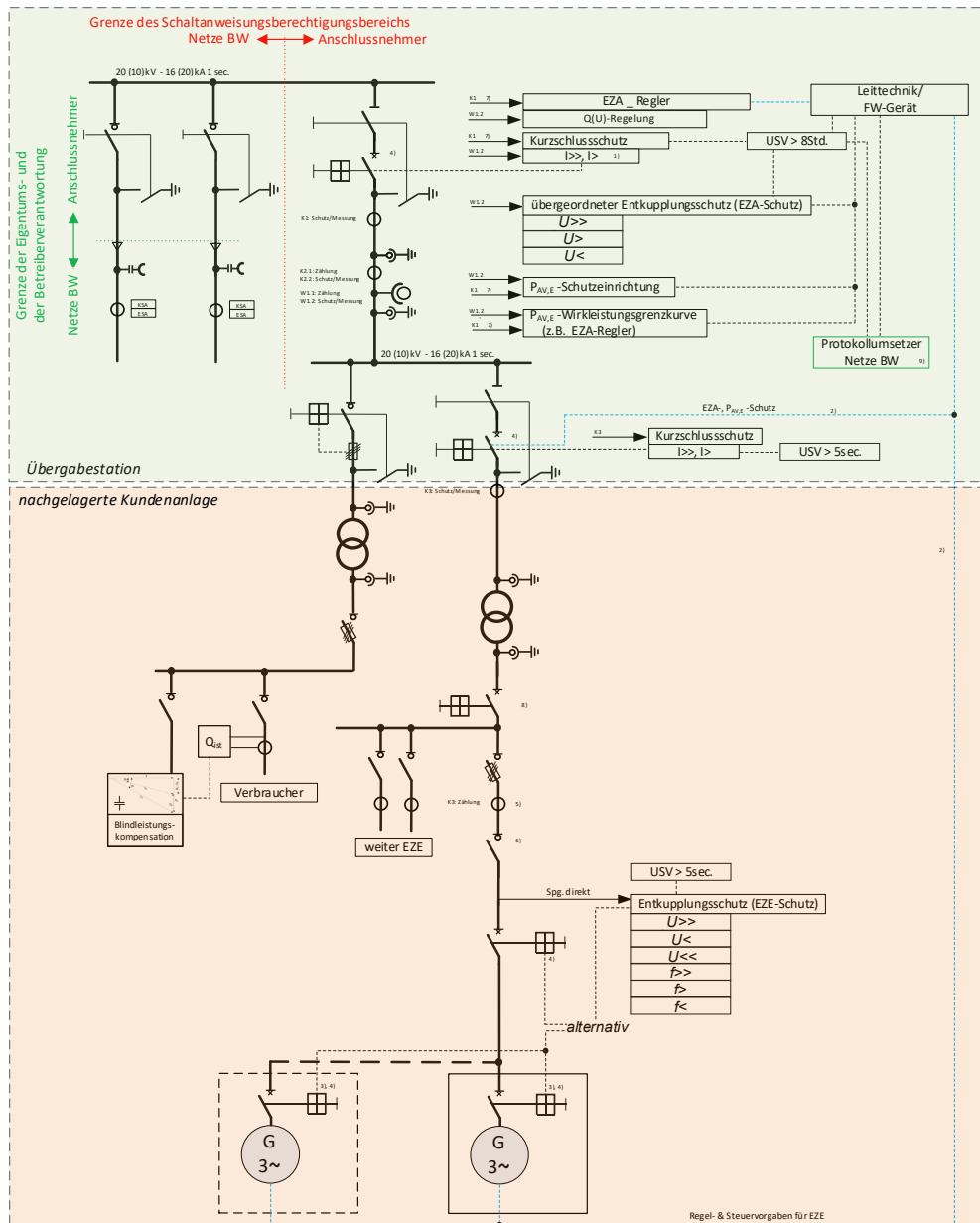
Bild D. 12: Misanlage mit Übergabeleistungsschalter und separatem Transformator mit Leistungsschalter für die Erzeugungsanlage ( \sum EZA > 950 \text{ kW} )
