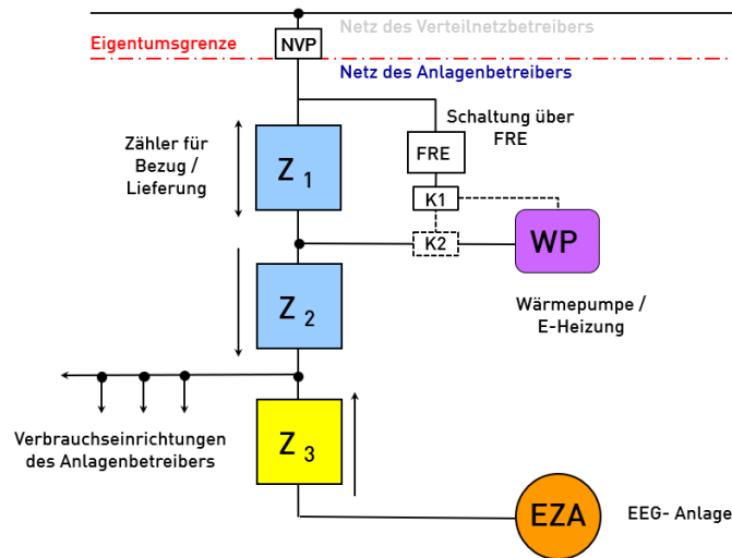
Abbildung 2: Gesteuertes Anschluss Wärmepumpe Kaskade inklusive Erzeugungsanlage
