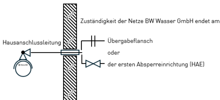
Abbildung 1: Übergabepunkt der Hausanschlussleitung
