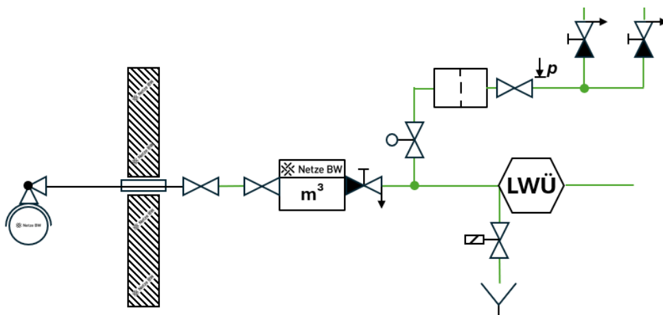
Abbildung 14: Darstellung einer Löschwasserübergabestelle
