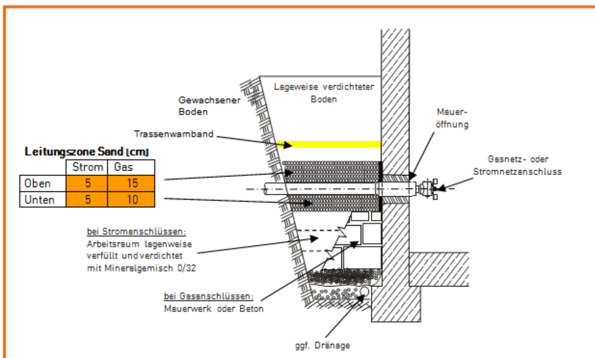
Abbildung: Unterbauung Netzanschluss im Bereich des Arbeitsraums
