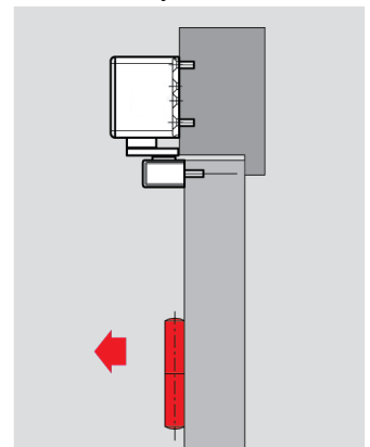
Kozijndorpelmontage scharnierzijde
