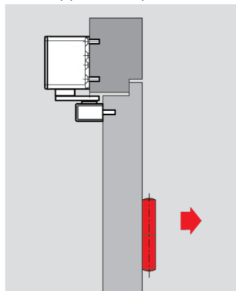
Montage renversé côté opposé aux paumelles
