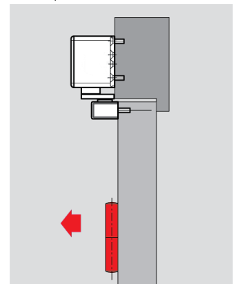
Montage renversé côté paumelles
