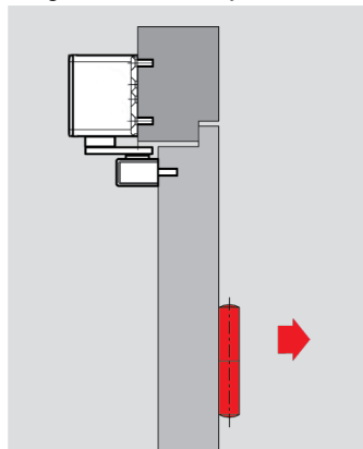
Kozijndorpelmontage tegenscharnierzijde
