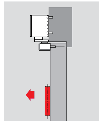
Kozijndorpelmontage scharnierzijde
