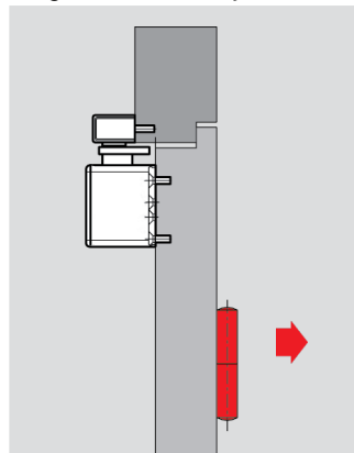
Deurbladmontage tegenscharnierzijde
