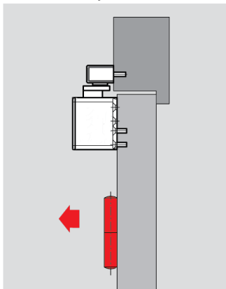
Deurbladmontage scharnierzijde
