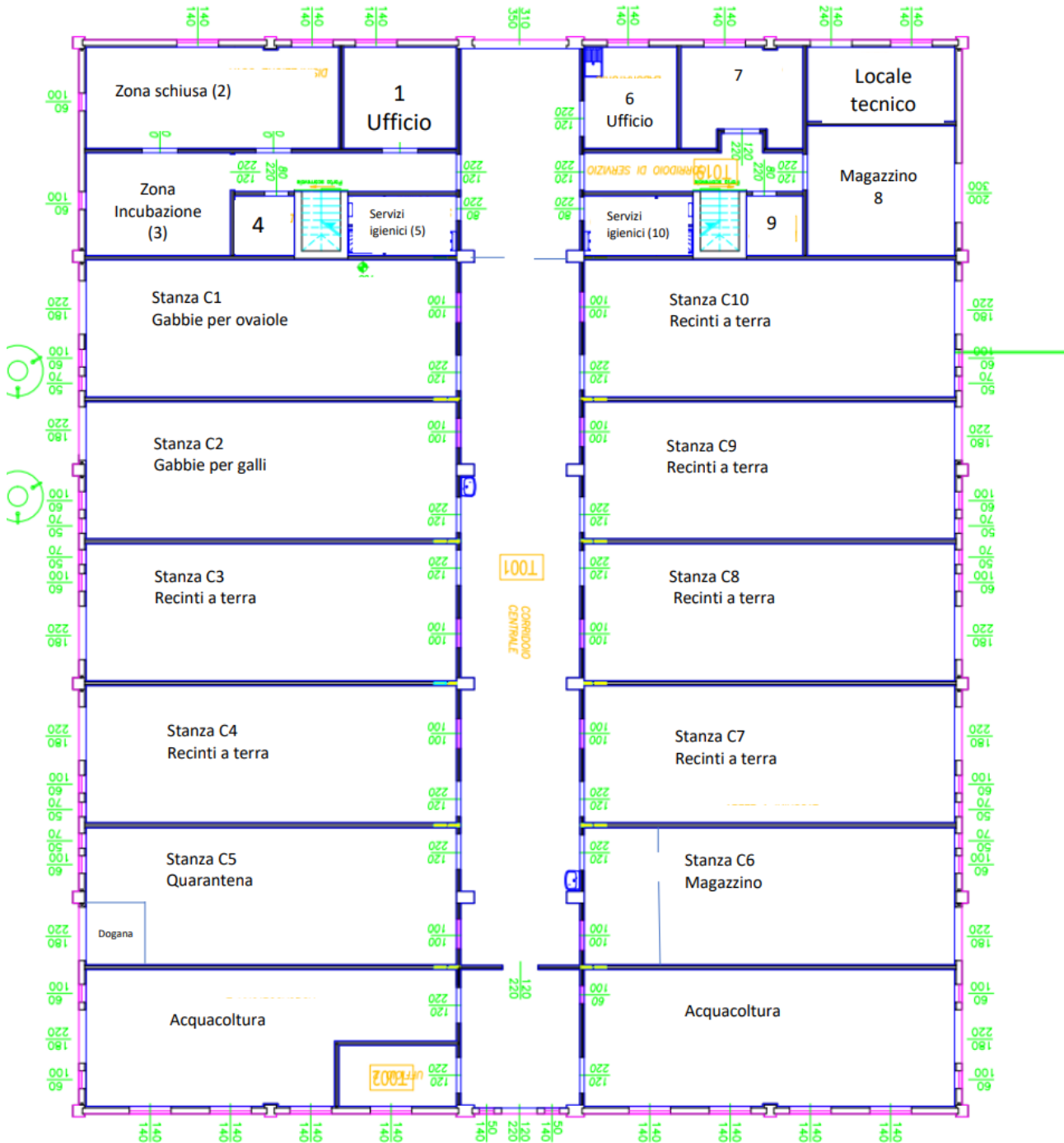
Allegato 2a– Planimetria edificio C Zoocolture con indicazione numero locale e destinazione uso
