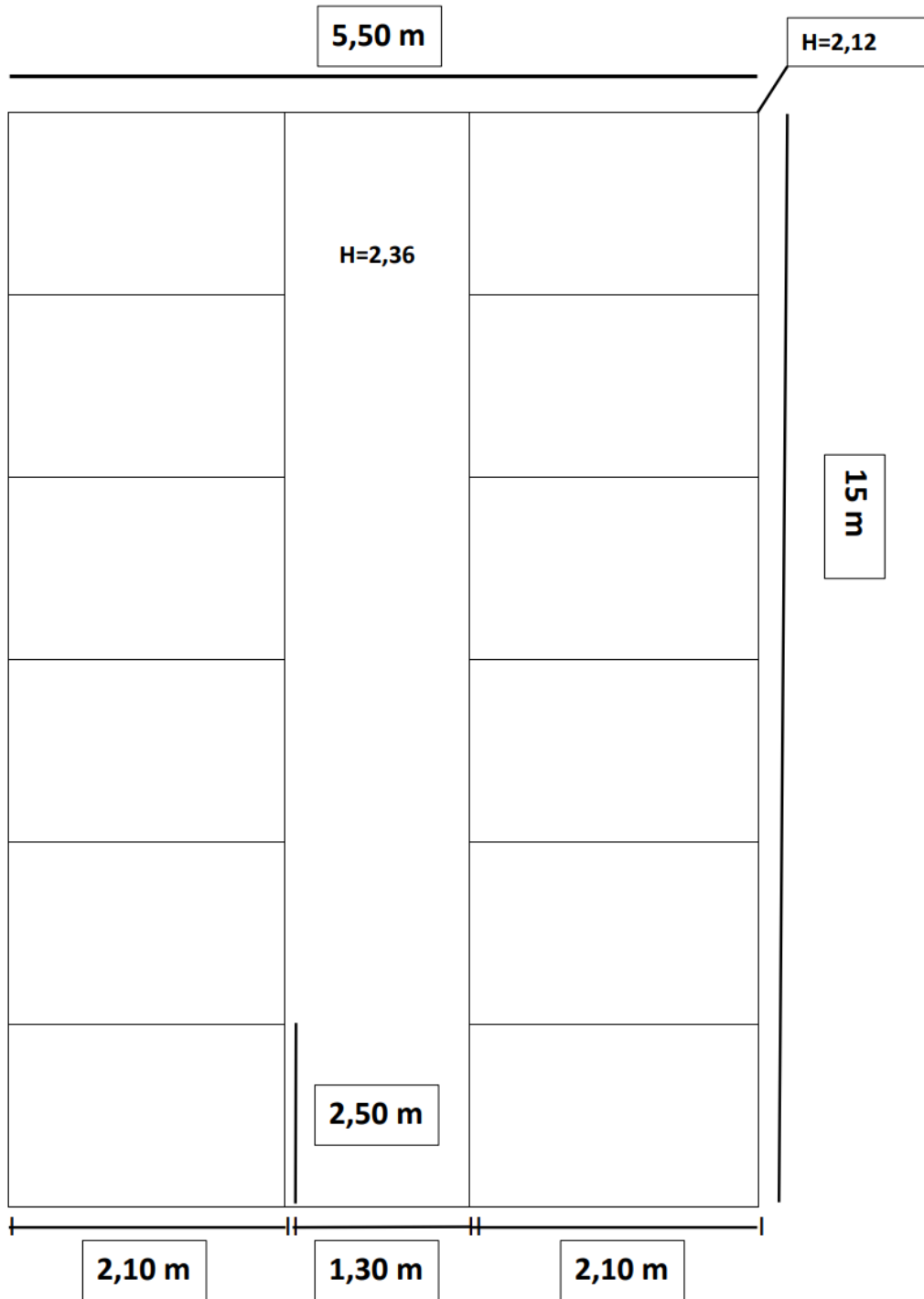
Allegato 2b – Planimetria recinti esterni edificio C- Zoocolture con indicazione delle principali misure
