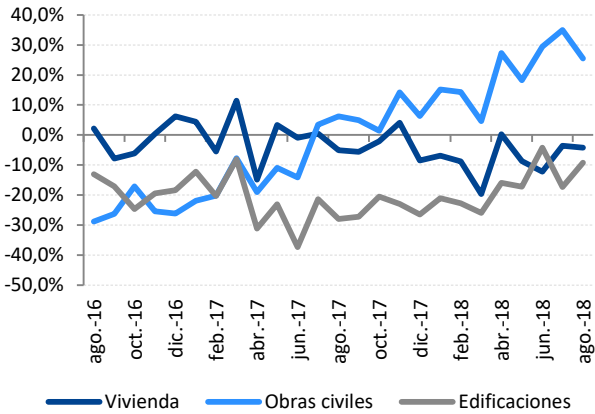
Gráfica 3. Producción de concreto por destino (var a/a)
