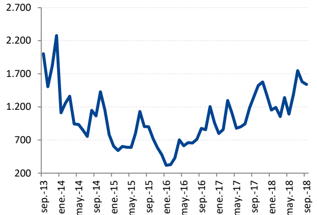
Gráfica 6. Baltic Dry Index (puntos)
