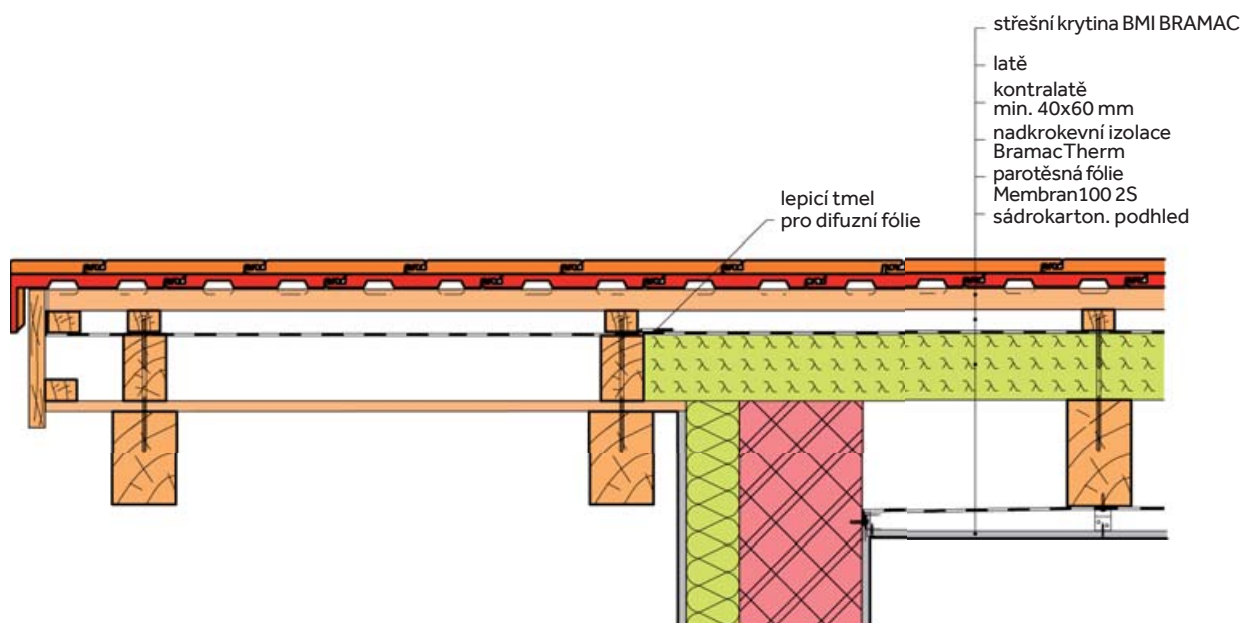
DETAIL ŠTÍTOVÉ HRANY S VELKÝM PŘESAHEM
