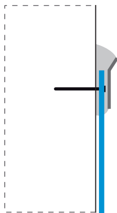
Ukončení pomocí přítlačné lišty - fólie je chráněna přítlačnou lištou
