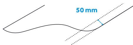
Minimální přeložení pro volně pokládané fólie stabilizované přitžením je 50 mm
