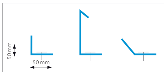
lišty pro kotvení do vodorovné konstrukce
