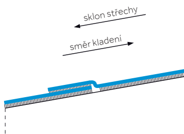
Minimální přeložení mechanicky kotvených fólií při použití podložek 40 x 82 mm nebo teleskopů je 110 mm
