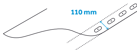
Minimální přeložení mechanicky kotvených fólií při použití podložek 40 x 82 mm nebo teleskopů je 110 mm
