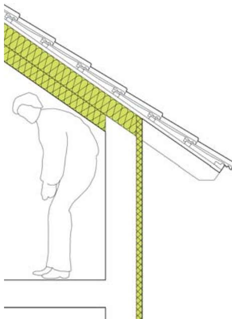
Obr. Standardní zateplení mezi a pod krokvy
