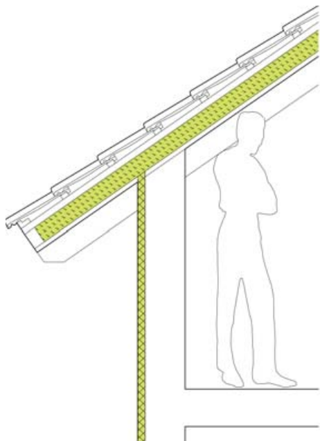
Obr. Zateplení izolací BramacTherm
