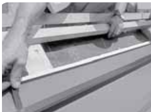
Montajul profilului din aluminiu
