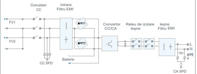
Schema circuitului
