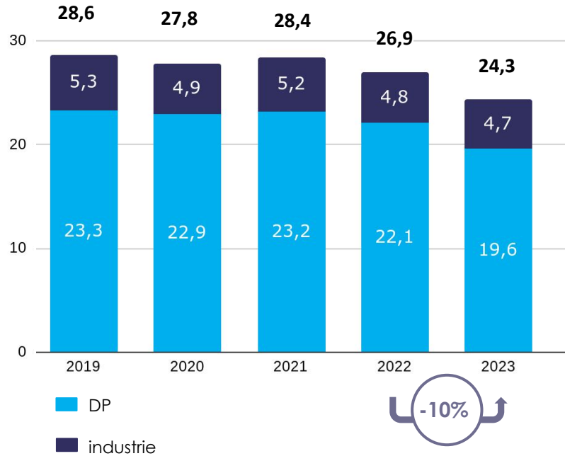
Évolution des consommations Teréga / corrigées du climat (TWh)
