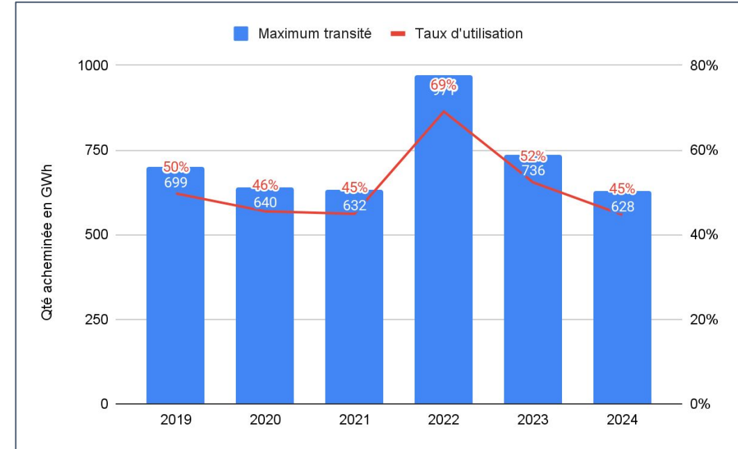
Quantités journalière maximum acheminées sur le réseau Teréga (2019 à 2024) et Taux d'utilisation par rapport aux capacités maximales du jour
