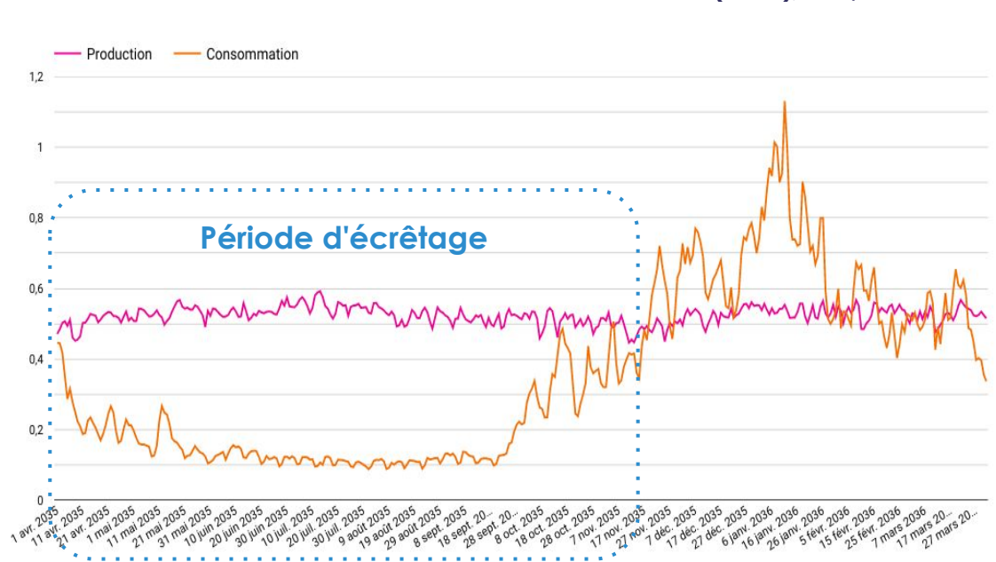
Consommation et production par zonage
