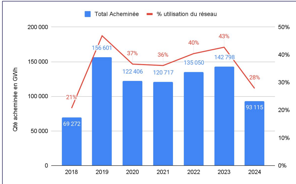
Quantités annuelles acheminées sur le réseau Teréga (2019 à 2024) et Taux d'utilisation par rapport aux capacités maximales
