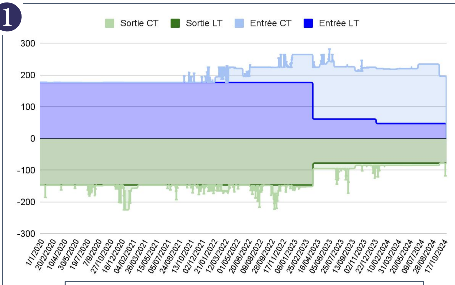
Souscriptions* au VIP Pirineos en GWh/j
